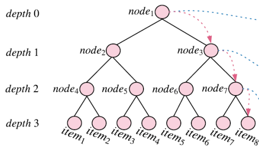
شکل ۴. ساختار درخت دودویی قبل از انجام خوشه‌بندی سلسله‌مراتبی [۲۳]
