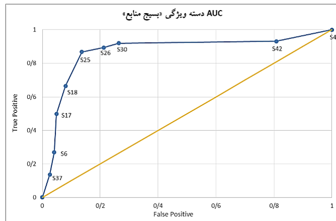
شکل ۱۰. نمودار ROC دسته ویژگی «بسیج منابع»
