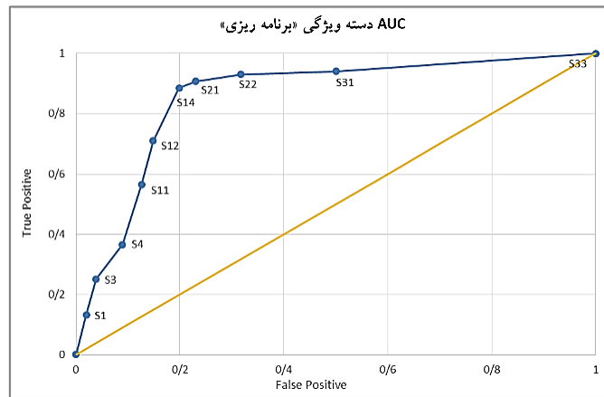
شکل ۹. نمودار ROC دسته ویژگی «برنامه‌ریزی»
