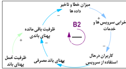
شکل ۲. حلقه B2 متعادل‌کننده پهنای باند مصرفی و کاربران.
