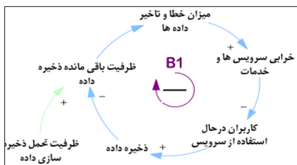
شکل ۱. حلقه B1 متعادل‌کننده ذخیره‌سازی اطلاعات و کاربران.
