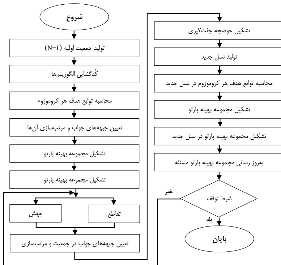
شکل ۲. فلوجارت نمایش مراحل الگوریتم فرآینتکاری NSGA-II
