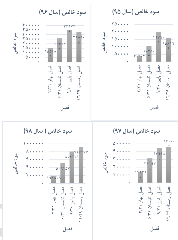
شکل (۶): پیش بردارزش اولیه داده های سود خالص در سال های ۹۵-۹۸
