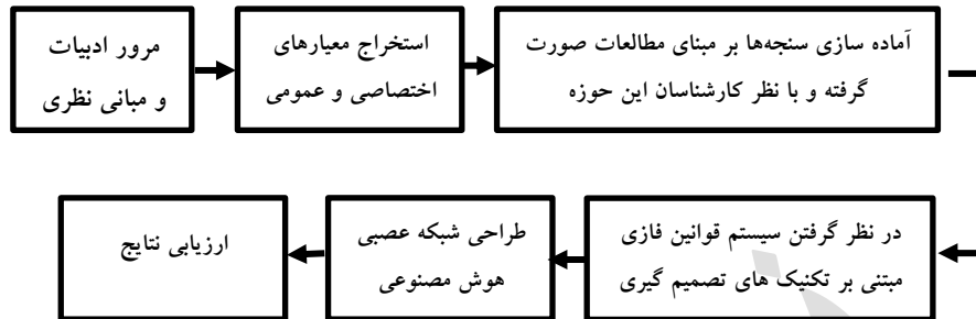
شکل (۱): فرآیند اجرایی تحقیق
