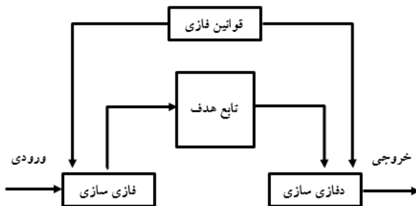
شکل (۲): ساختار سیستم فازی در الگوریتم به کار رفته [۱۸]
